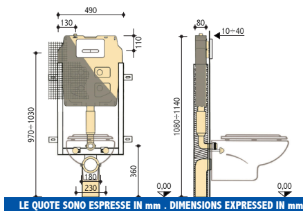
LE QUOTE SONO ESPRESSE IN mm . DIMENSIONS EXPRESSED IN mm
